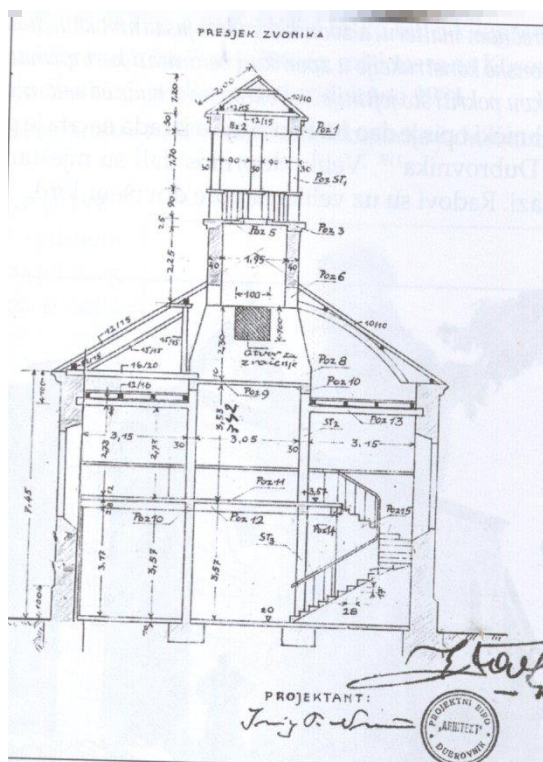
Slika 6. Poprečni presjek na prednjem dijelu sa zvonikom
